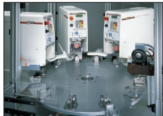
Modul mit 3 Hermetic 6-11 und drehbaren Werkstückaufnahmen
